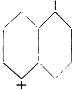
L Säure. Erdmann. Annal. 247. 343. Schulz. Ber. 20. 3161.
